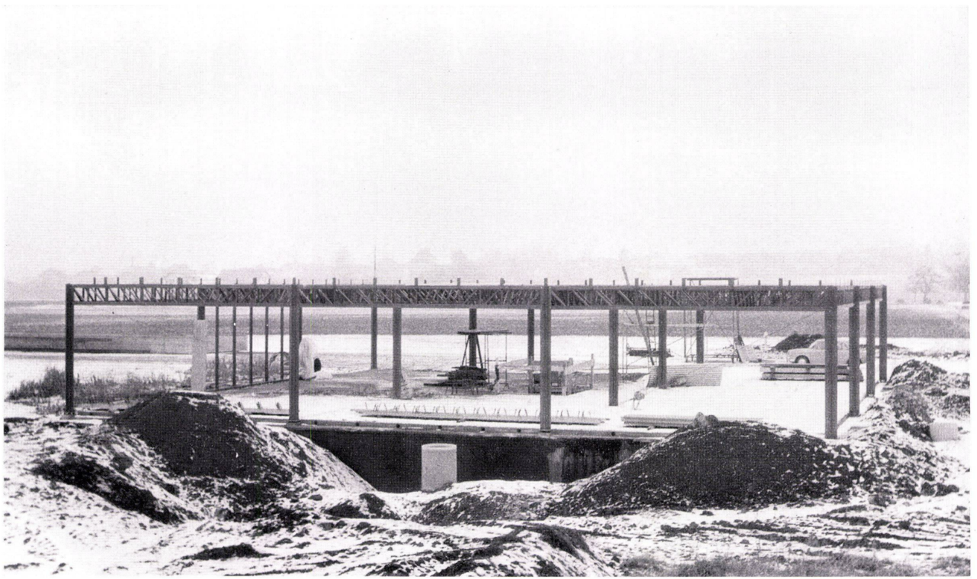
1 Fertig montiertes Stahlgerüst. Echafandage en acier, complètement montée. Steel structure scaffolding, completely mounted.
