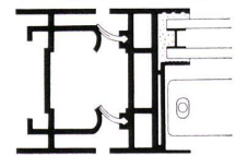
Rotationsfenster mit Lippendichtung
