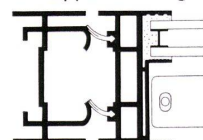
Rotationsfenster mit Lippendichtung
