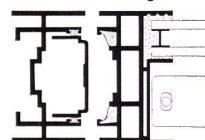
Rotationsfenster mit Schließzunge
