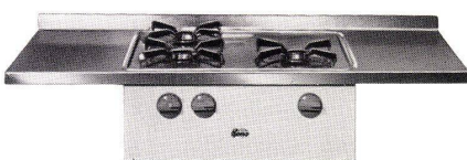
Einbau-Kochtisch, Modell 733 zum Einbau in Spültischkombinationen, Abdeckung aus Chromnickelstahl mit verlängerten Abstellflächen. 1 Starkbrenner, 2 Normalbrenner; gelenkige, rost sichere Pfannenträger
