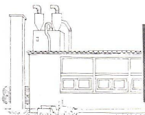
Zentralheizungskessel 600: Wechselbrand, jedem Wunsch anpassbar. 45 Typen für 120000 bis 1400000 kcal/h.
