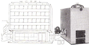
Zweistoff-Zentralheizungskessel 1100: Einzigartig für geruchlose Kehricht-Verwertung. 15 Typen für 100000 bis 1200000 kcal/h.
