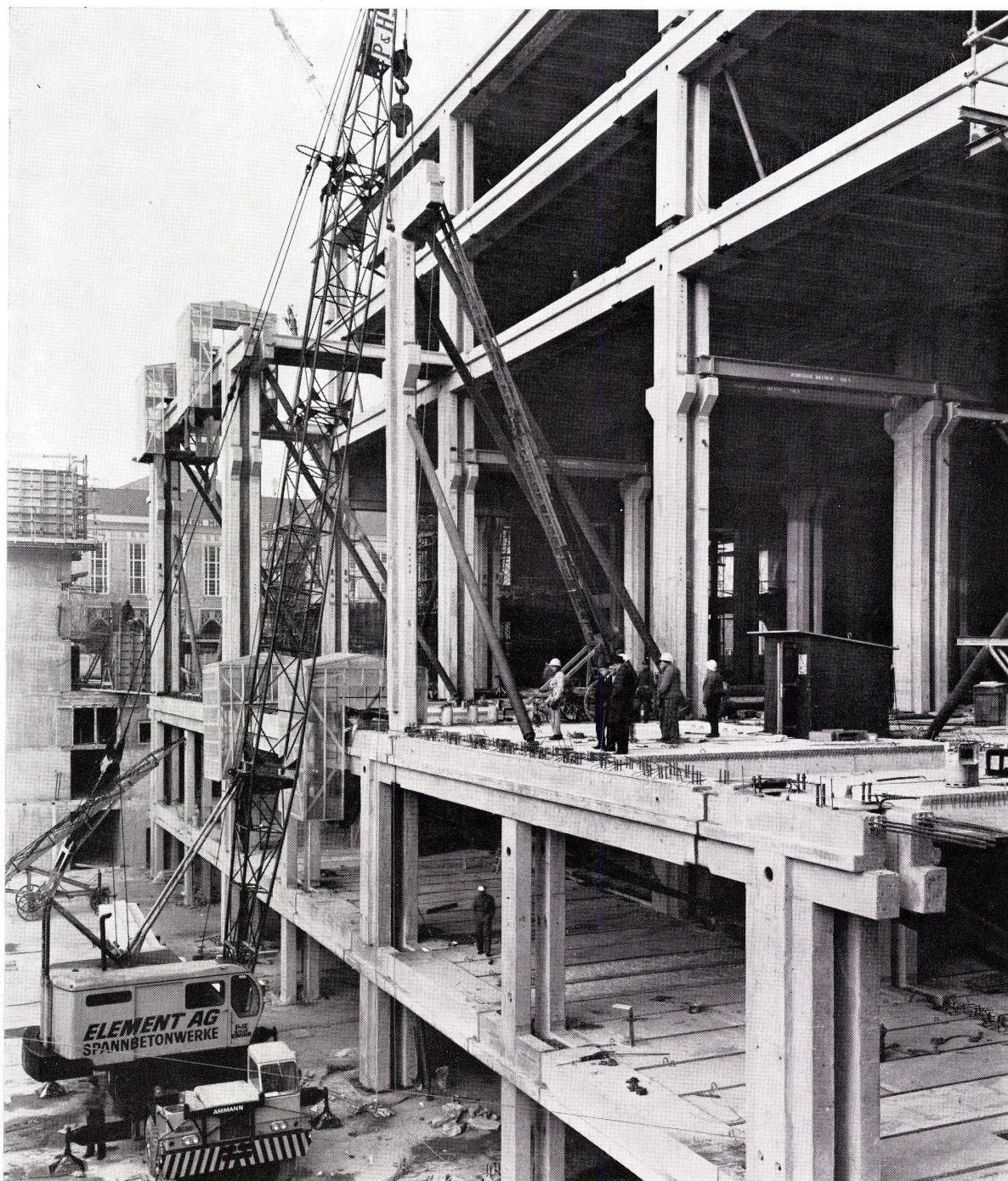
Mustermesse Basel, Hallenneubau Rosental, Basel. Montage der vorfabrizierten Hallenkonstruktion
