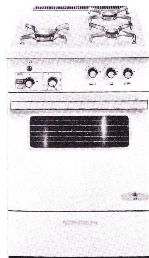
MENA-LUX/ARTHUR MARTIN 543 Luxusmodell mit 3 Kochstellen. Backofen mit Schauglas, Innenbeleuchtung und Infrarotgrill, auf Wunsch mit elektrischem Drehspeiß erhältlich. Zündsicherung für Grill und Backofen. Normierte Dimensionen: 55/60/85. Höhe nach Wunsch auch 90 oder 80
