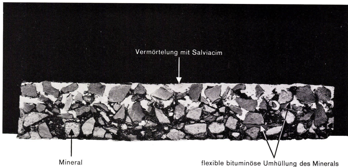
Belags-Querschnitt einer Salviacim-Deckschicht, Körnung 0/10 mm
