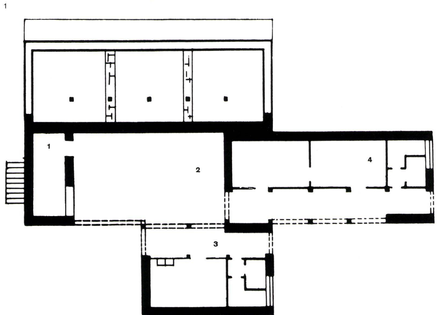
2 1 Obergeschoßgrundriß Garderobengebäude 1:200. Bâtiment vestiaire, plan d'étage supérieur. Upper floor plan dressing-room building.
