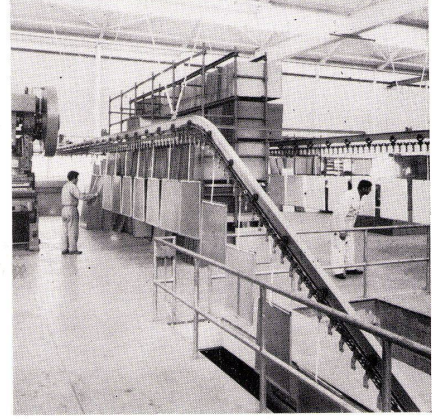
Teilansicht aus der Lackieranlage
