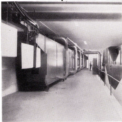
Tunneleinbrennofen in der Lackieranlage
