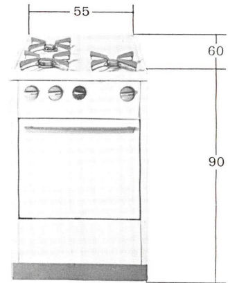
Genormte Abmessungen 55/60/90. Höhe variabel nach Wunsch 80+85.
