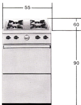
Normierte Abmessungen 55/60/90 Höhe variabel nach Wunsch 80+85
