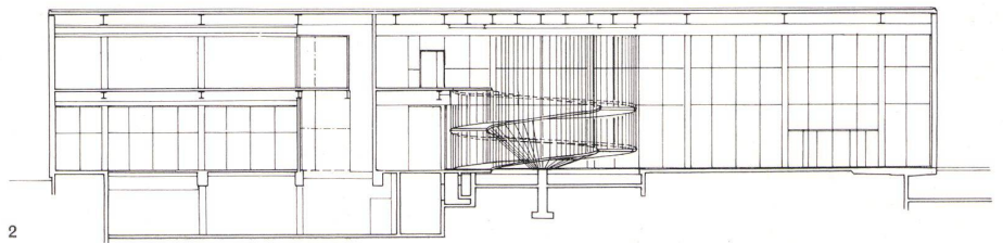
2 Zentrale Eingangshalle mit gewendelter Rampe 1:300. Hall d'entrée central et rampe d'accès. Central lobby with spiral ramp.
