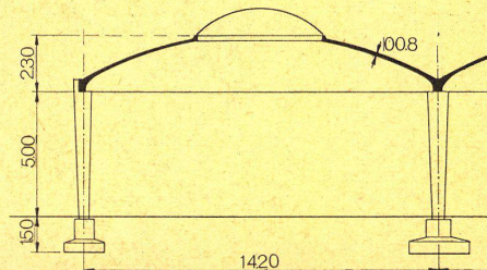
5 Schnitt durch eine Buckelschale in Spannbeton von 14 x 20 m, mit einer Großlichtkuppel von 5 m Durchmesser. Eschmann AG, Thun.
