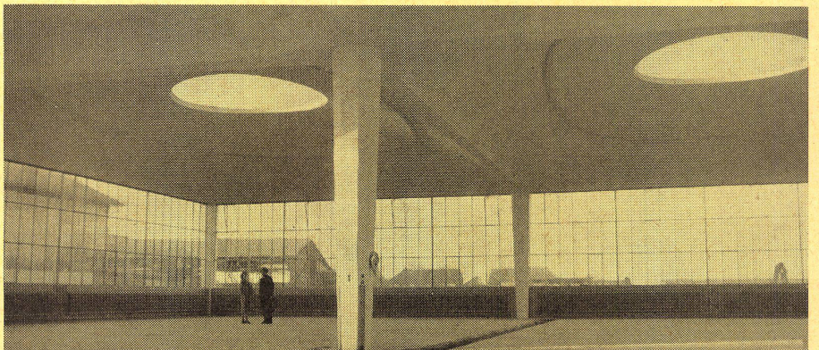
3 15 auf Ecken abgestützte Buckelschalen. Wollspinnerei Huttwil. Projekt: Weder und Prim, Ing. Langenthal. Mitarbeiter für Buckelschalen H. Isler, architektonische Beratung: Lüscher und Clavadetscher, St. Gallen. 15 coquilles bombées portées dans les coins. Filature de laine Huttwil.
