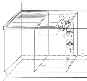
Beispiel mit Kunststoff-Ablaufinstallation mit Bögen, T-Stück und Syphon
