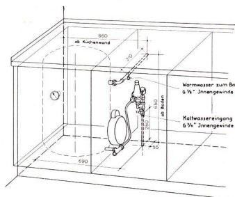
Hydraulische Installation des Boilers Becken-Ablaufinstallation
