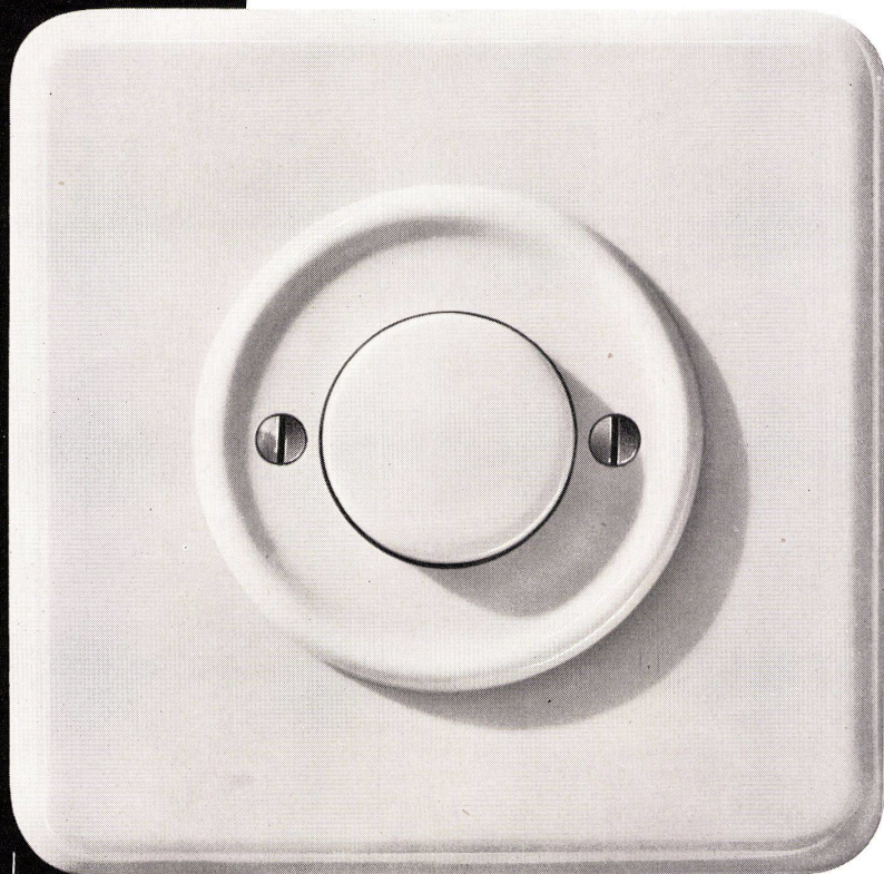
Druckknopfschalter 10 A 380 V ~
