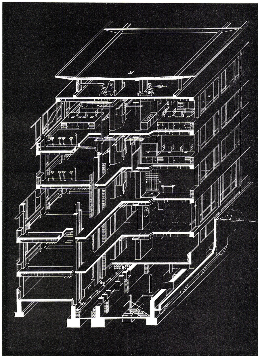
2 Isometrie mit Darstellung der Konstruktion, Leitungsführung und Einrichtung. Isométrie montrant la construction, les conduites et l'installation.
