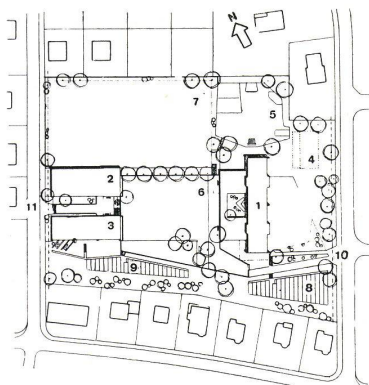
Situation / Site 1:2500
