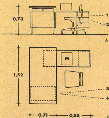
A Ansicht B Grundriß
