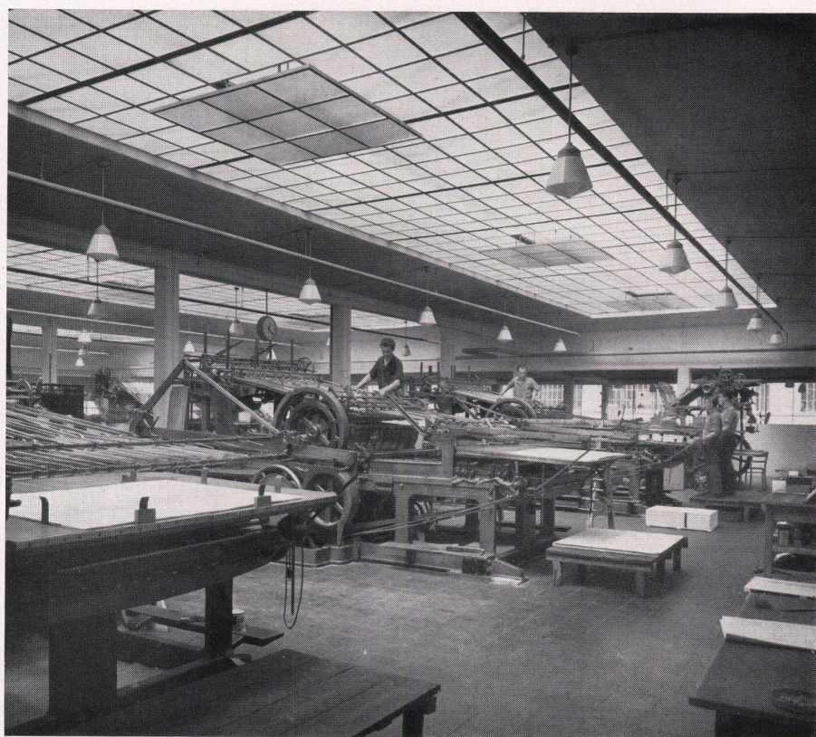
Druckereisal im Erdgeschoß. Salle d'impression au rez-de-chaussée. Printing room on ground-floor.
