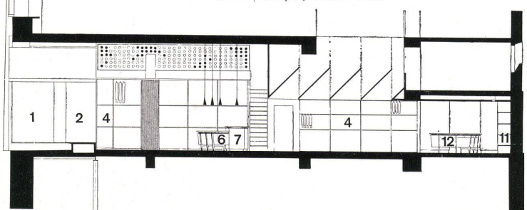
Schnitt / Coupe / Section 1:200
