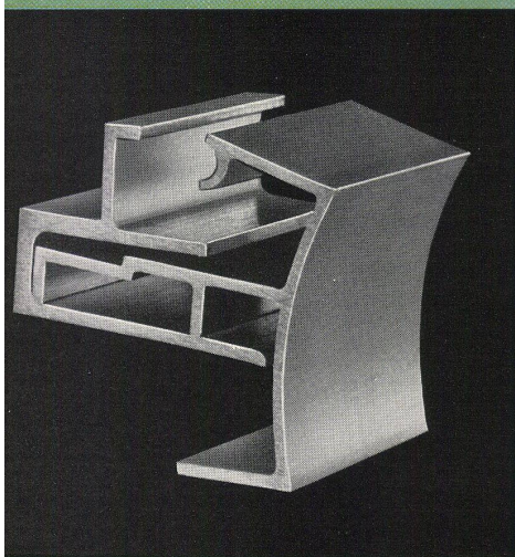
Sessa-Schaufenster-Rahmen-Konstruktion
