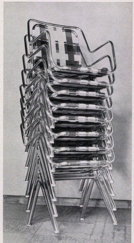
Stapelbarer Armsessel auf Bockbeinen in rostfreiem Duraluminium. Sitzteil beweglich auf Beinen montiert. Nylongurten.
