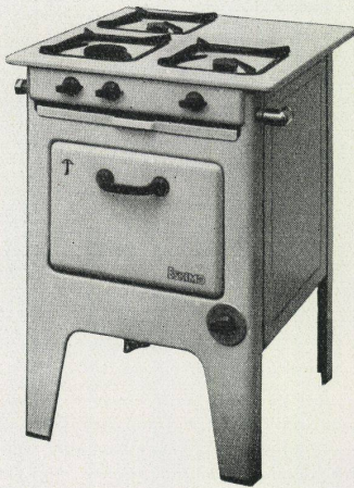
3 Kochstellen mit Brat-Grill, Backofen mit Temperatur-Regler / Höhe des Herdes 800 mm / Kochplatte 585 x 585 mm / Gewicht zirka 53,4 kg.
