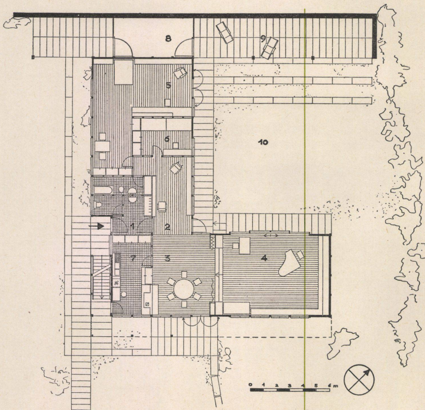
Erdgeschoß / Rez-de-chaussée / Ground floor 1 : 250
