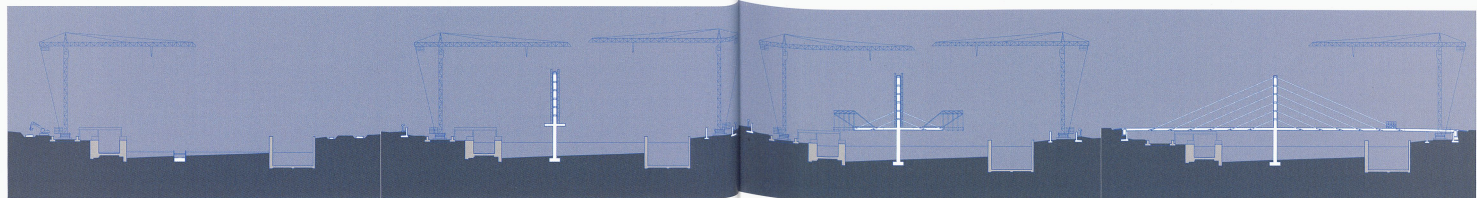
2 Coupe du pont existant, de la pile centrale du futur ouvrage d'art, du futur tablier et coupe du barrage de dérivation 3 a. Efforts normaux dans le tablier [kN] b. Moments de flexion dans le tablier [kNm] c. Efforts tranchants dans le tablier [kN] 4 Phase de construction du futur pont
