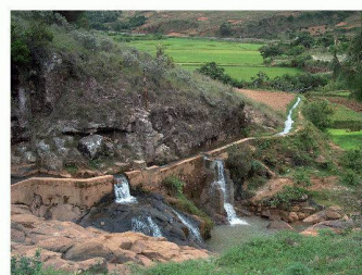
Site d'implantation pour une pico-centrale (Photo AZ Ingénierie)
