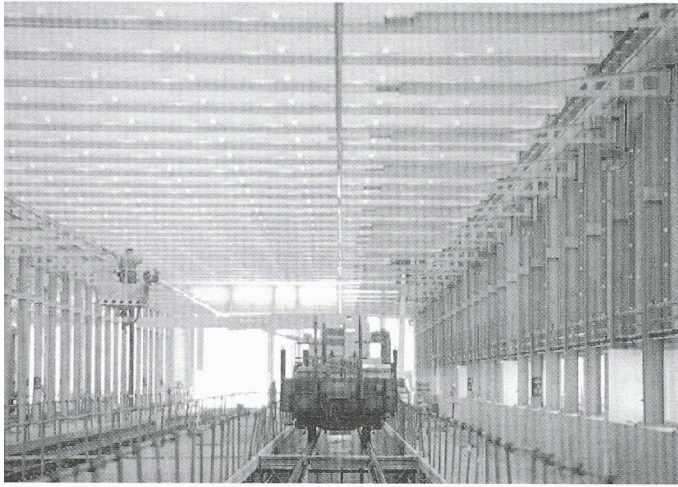
Fig. 2.- Assemblage du système (Photo Furrer+Frey)
