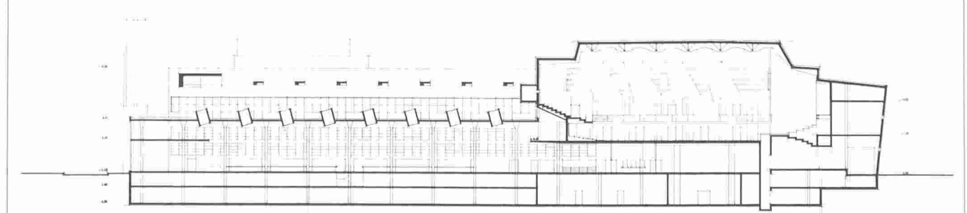
Coupe longitudinale
