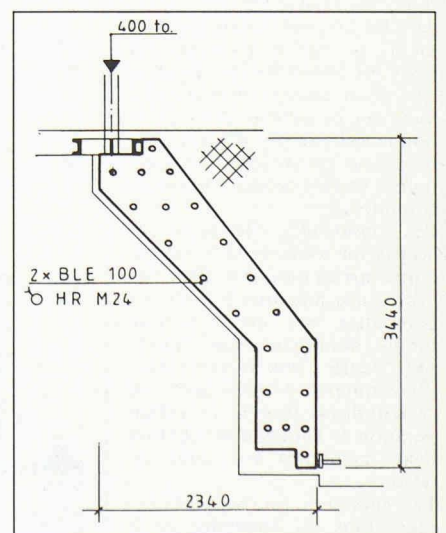
Fig. 13. — Béquille inclinée à section pleine.
