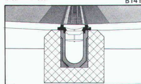
2ème phase: l'élément surélevé est posé sur le caniveau. Maintenant le revêtement définitif peut être mis en place et compacté jusque contre le caniveau.
