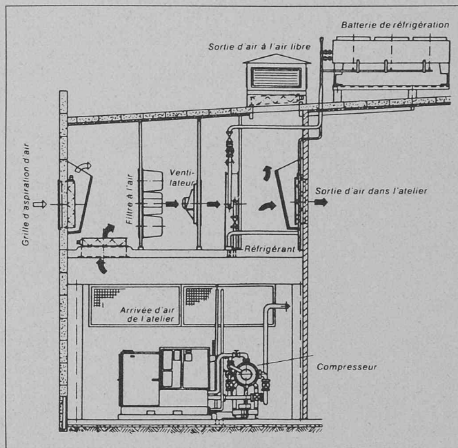
Fig. 3. — Schéma de principe d'un compresseur refroidi à l'eau.
