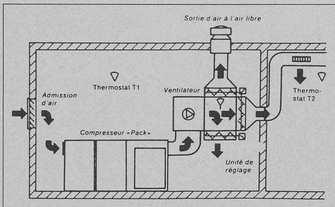
Fig. 1. — Schéma de principe d'un compresseur refroidi à l'air avec récupération de chaleur. Utilisation directe de l'air de refroidissement réchauffé pour le chauffage de locaux.
