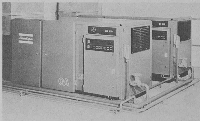
Installation d'un compresseur GA-Pack avec conduits d'air pour la récupération de chaleur.
