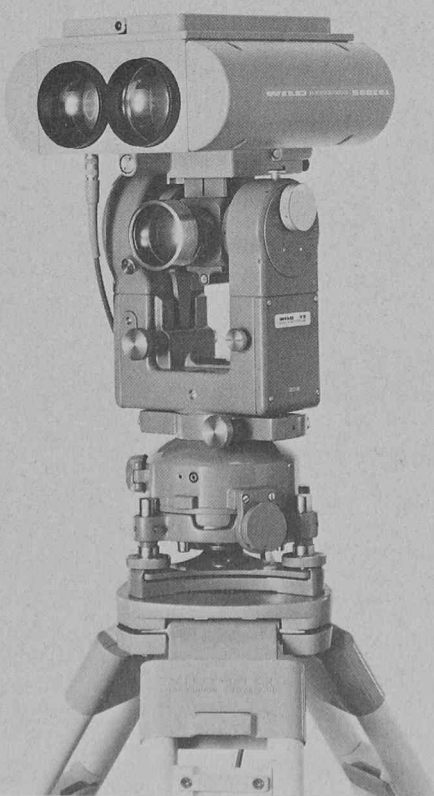
Wild Distomat DI20 sur théodolite universel Wild T2.
