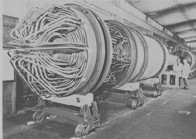
Vue d'un générateur de vapeur d'un réacteur au thorium à haute température du côté entrée de l'hélium. Au premier plan, faisceau de resurchauffeur avec tubes de liaison; à l'arrière-plan, faisceau de surchauffeur.
