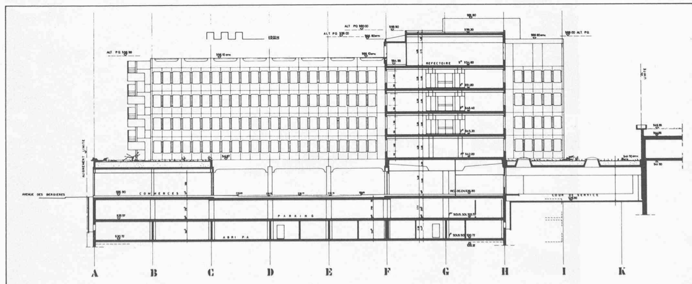
Fig. 4. — Coupe A-A.
