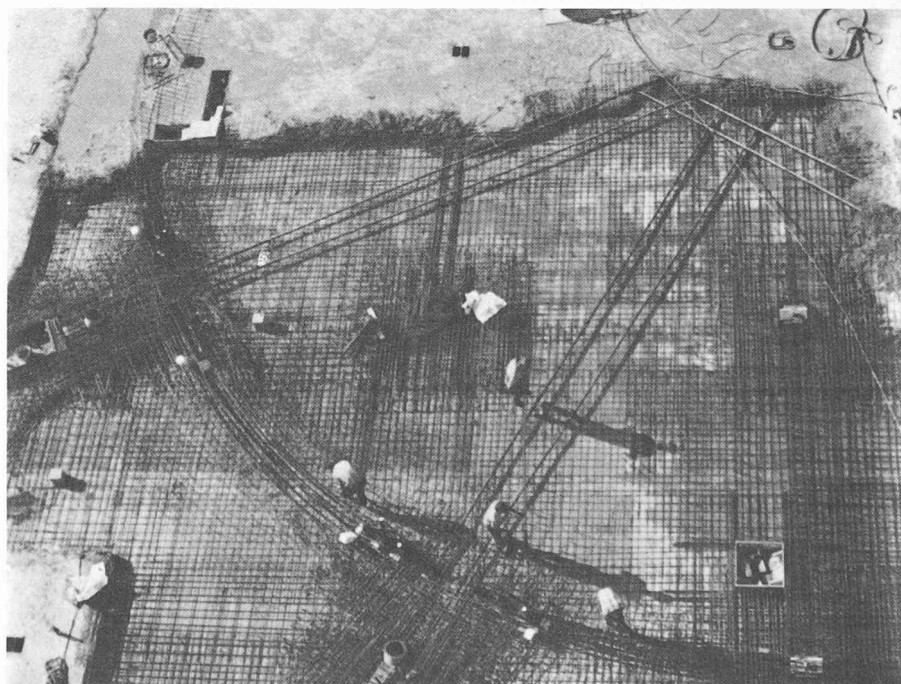
Armature et câblage du support de l'anneau circulaire.
