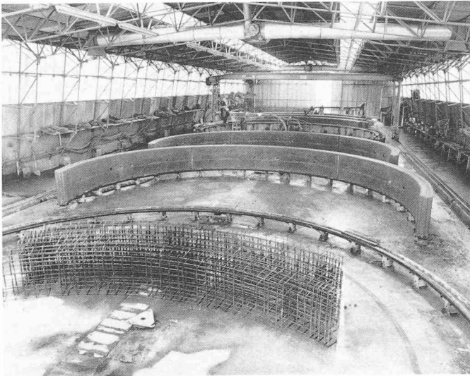
Fig. 3. — Lot ouest. Fabrication des voussoirs en béton près du point d'attaque médian
