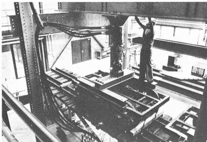
Mise en charge d'un pont de chemin de fer en vue d'un essai de fatigue (photo Foetisch).
