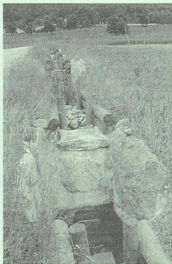
Bassin rétention-infiltration
