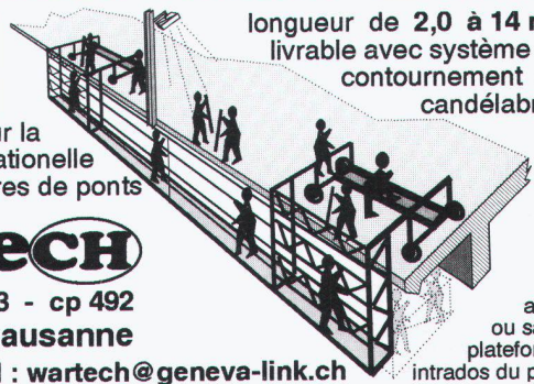
"CROC" avec train de roulement à emprise minimale sur les bords de la chaussée du pont
