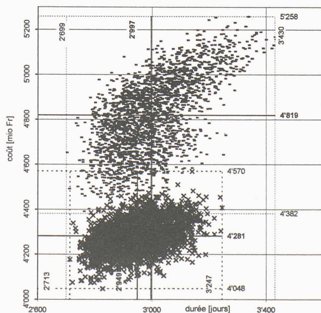
Fig. 2.- Diagramme temps-coûts du génie civil pour le tunnel de base du St-Gothard. Le nuage du bas (x) correspond à la variante actuellement confirmée quant à la composition de la zone de Piora au niveau du tunnel.
