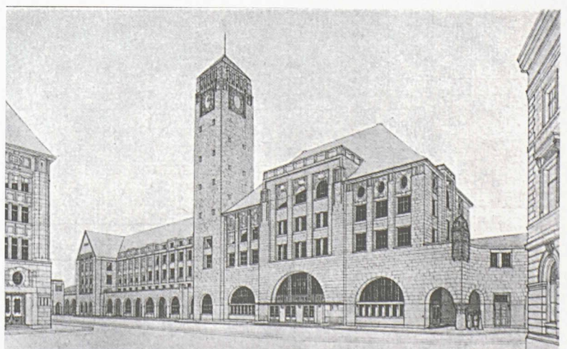
La gare de Saint-Gall, vue par les auteurs de l'un des trois projets ayant obtenu le 2 e prix ex aequo en 1908, soit Pflögard et Haefeli, architectes, Zurich. Il n'a pas été discerné de 1 er prix, «aucun des projets n'aurait pu être utilisé tel quel pour l'exécution des bâtiments».
