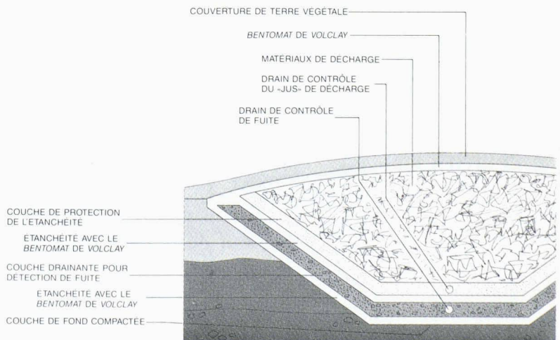
Etanchéité d'une décharge: schéma de principe
