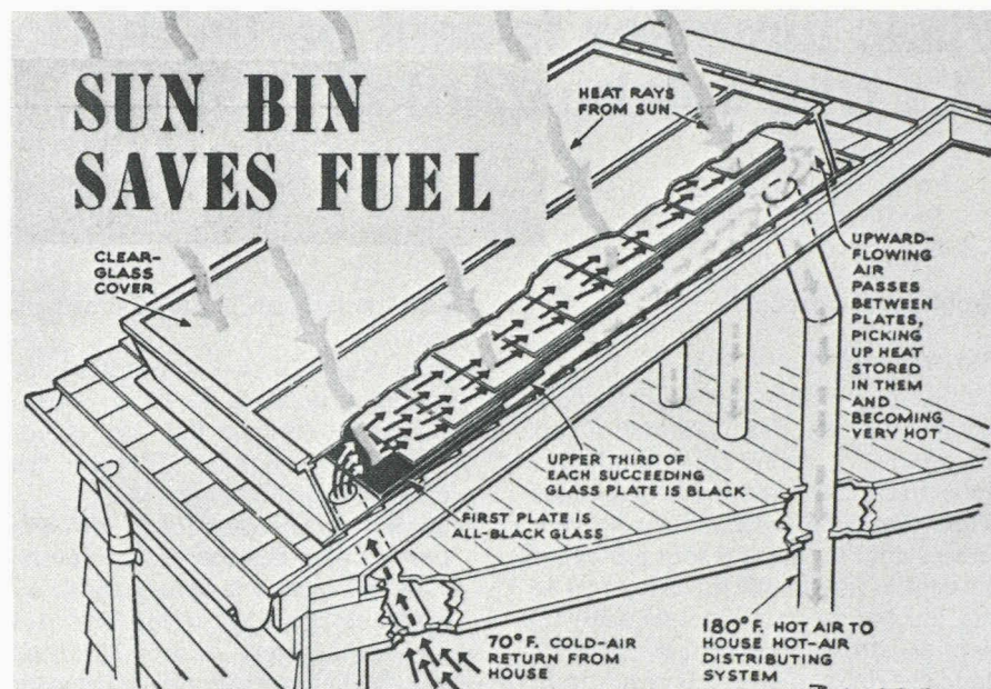
Fig. 3. - Système de chauffage solaire à air selon George Löf, Boulder, Colorado, 1930.
