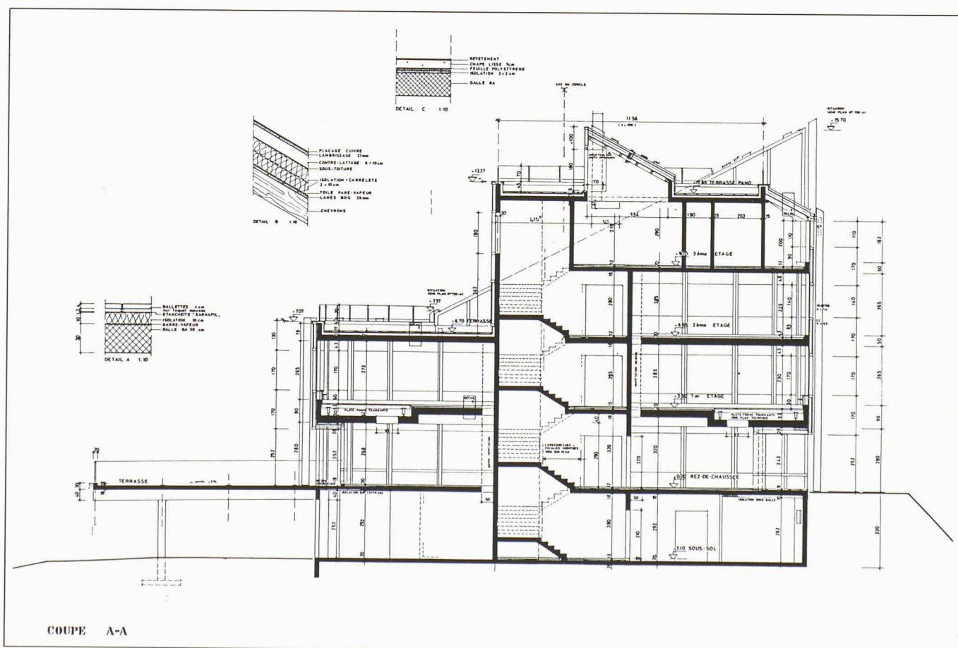
Fig. 3. - Coupe.
