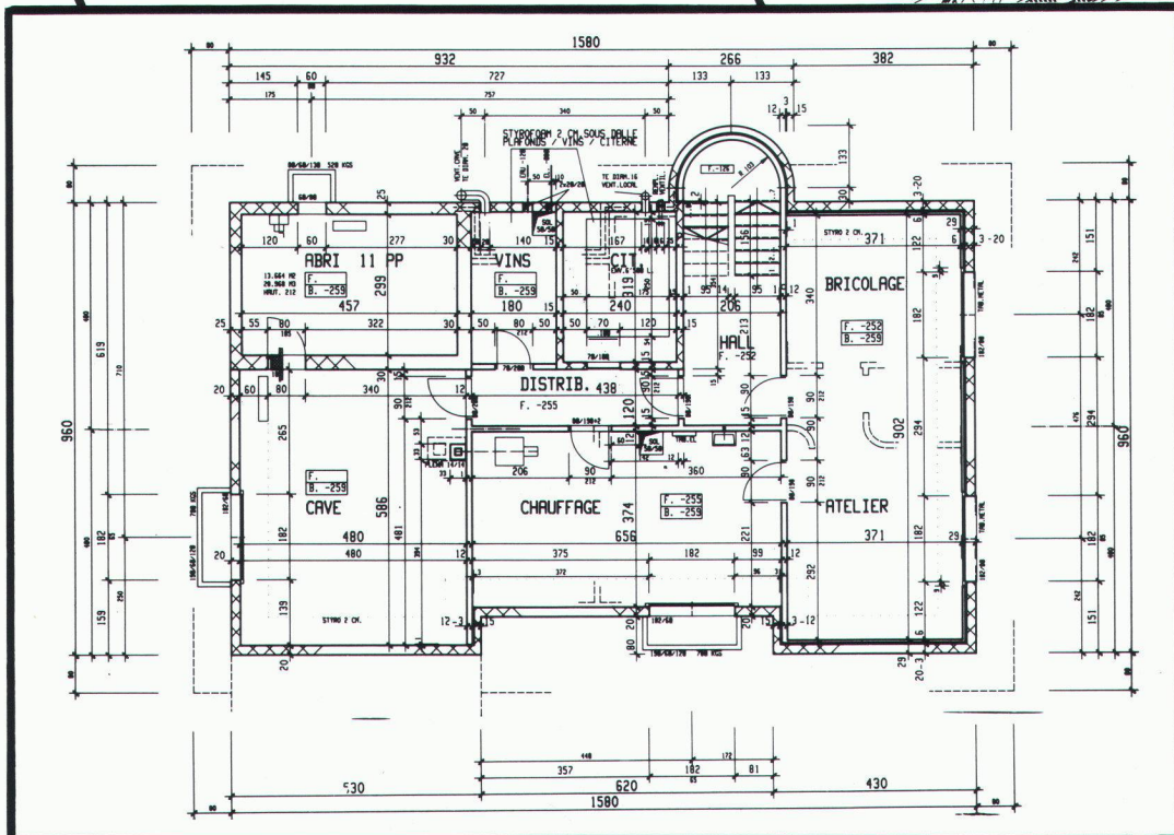
Exemple de plan réalisé avec la DAO ANNIE .
