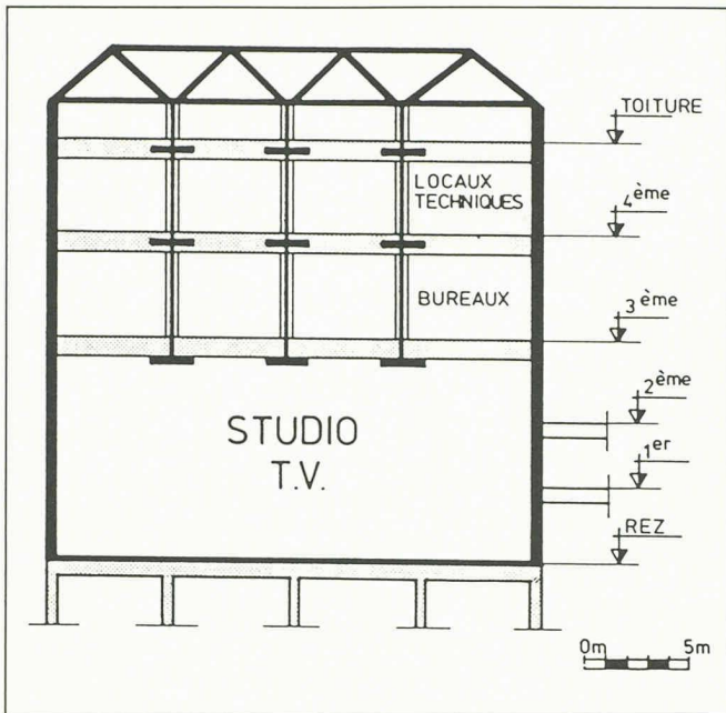
Fig. 1. - Coupe schématique du studio.
