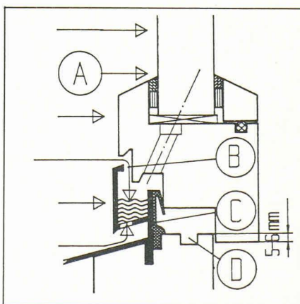
Fig. 3. — Evacuation de l'eau de pluie. A: Pression du vent. B: Joint de décompression. C: Étanchéité centrale. D: Rainure pour les ferrants.
