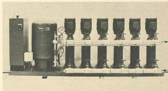
Surpresseur automatique Biral DWA-P commandé par microprocesseur pour l'amortissement des coups de béliet dans les réseaux fortement sollicités.
