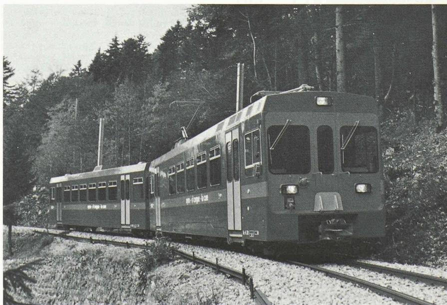
La première rame-navette, composée de l'automotrice Be 4/4 201 et de la voiture-pilote Bt 301, en service entre La Cure et Saint-Cergue. Elle représente l'unité de base pour les trains horaires. Grâce à leurs deux cabines de conduite, les automotrices peuvent aussi circuler seules. La possibilité de conduite en unités multiples par un seul agent, permet à un train comportant deux motrices et quatre voitures de transporter 896 personnes, dont 436 en places assises. (Photo BBC.)
