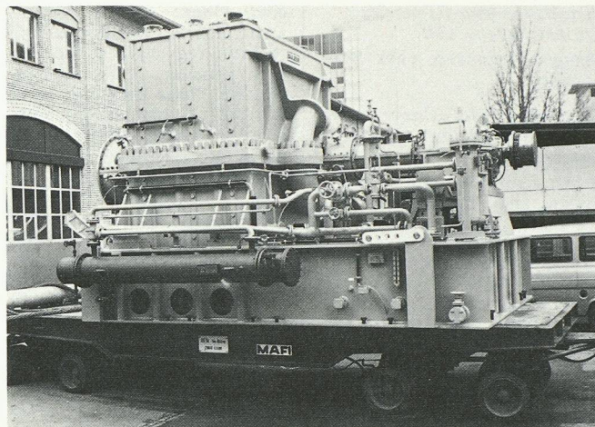
Compresseur isotherme Sulzer, type RIK 56.
