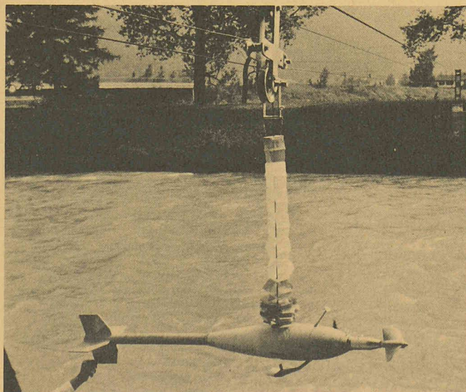
Le moulinet, fixé sur la partie droite du saumon, tourne à une vitesse qui est fonction de la vitesse de l'eau. Le saumon, muni d'ailerettes stabilisatrices, permet d'immerger et de stabiliser le moulinet dans le cours d'eau à l'endroit désiré. Les impulsions produites par le moulinet et le détecteur de fond (visible sous le saumon) sont transmises en surface par un câble électrique.
