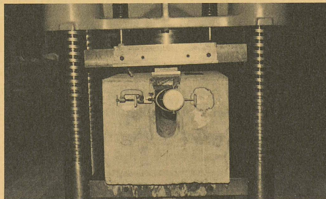
Fig. 3. — Polydrain enrobé de béton, sous la presse, charge verticale.
