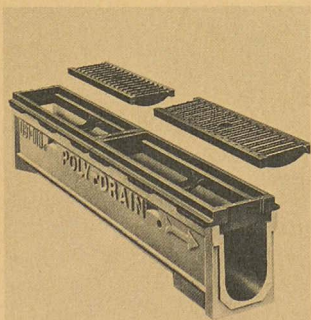
Fig. 1. — Le caniveau Polydrain en système Poly-Monofonte .
