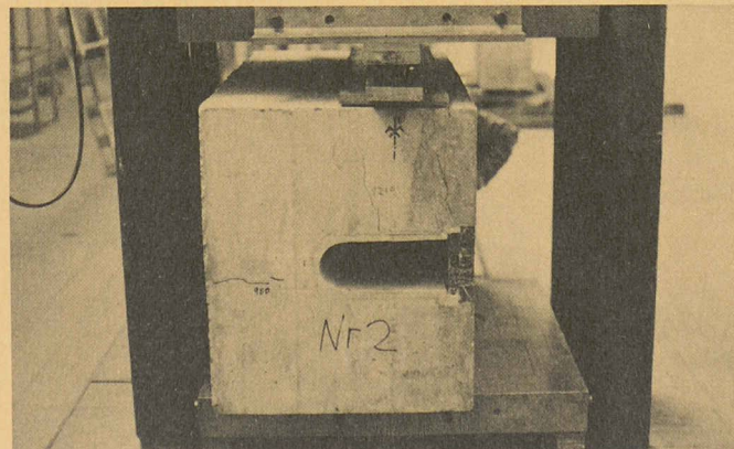
Fig. 4. — Polydrain enrobé de béton, sous la presse, charge horizontale.
