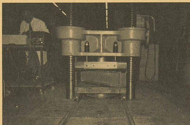
Fig. 2. — Caniveau reposant librement sous la presse.
