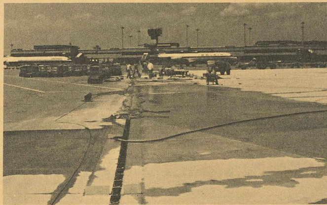
Fig. 5. — Polydrains posés dans du béton armé.
